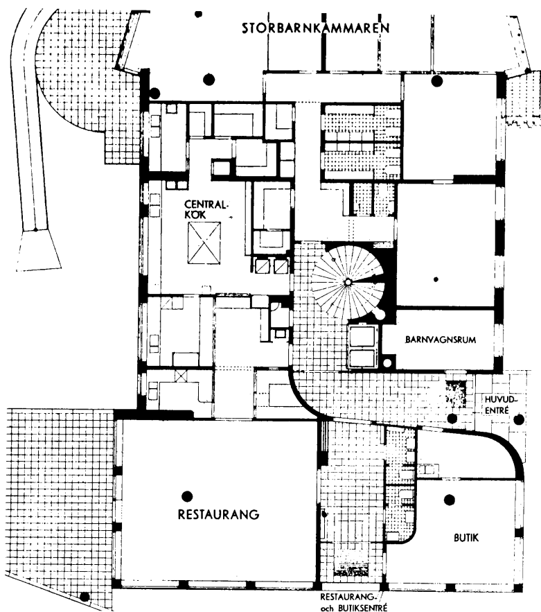
Plan av bottenvåningen i YK-huset.
