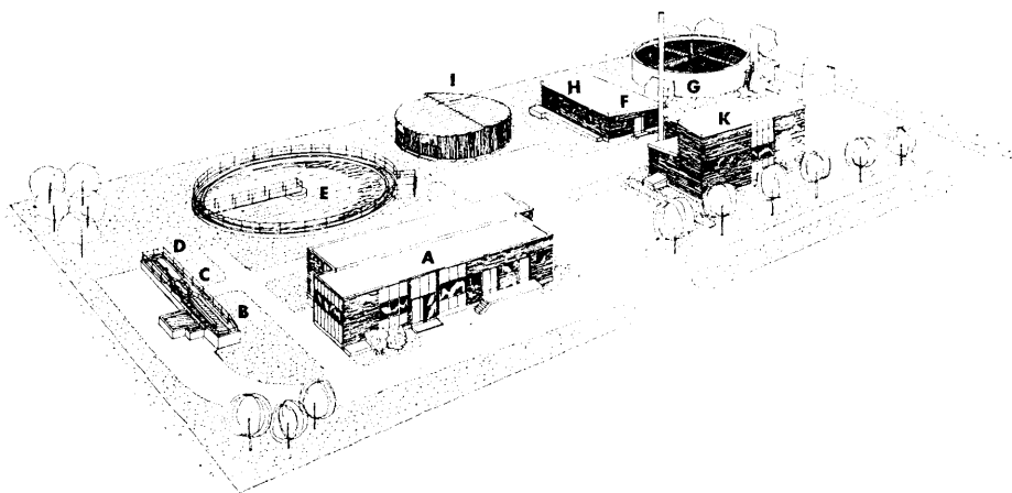
Kungsörs avloppsreningsverk (perspektivskiss).
