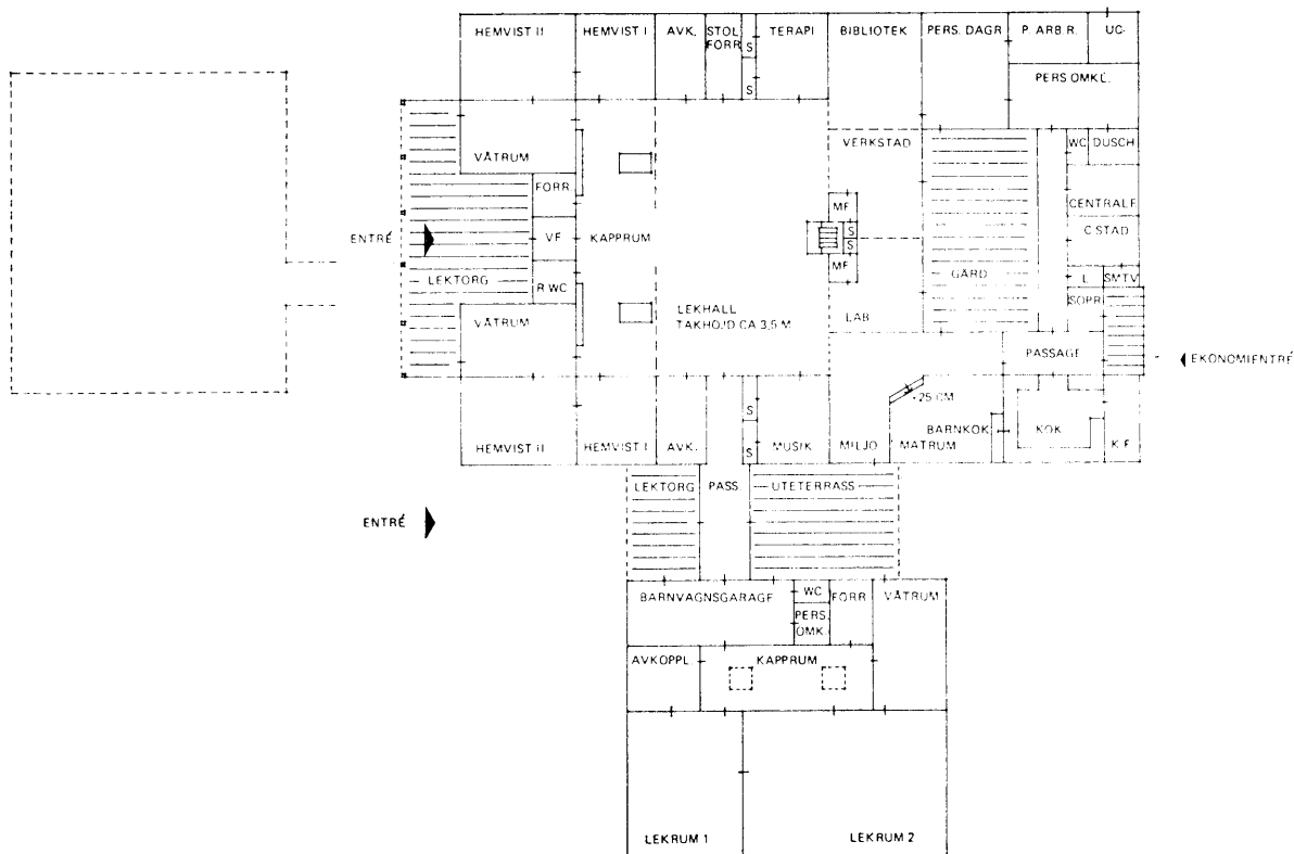
Planskiss på en framtida förskola. Hämtad ur Barnstugeutredningens PM.
