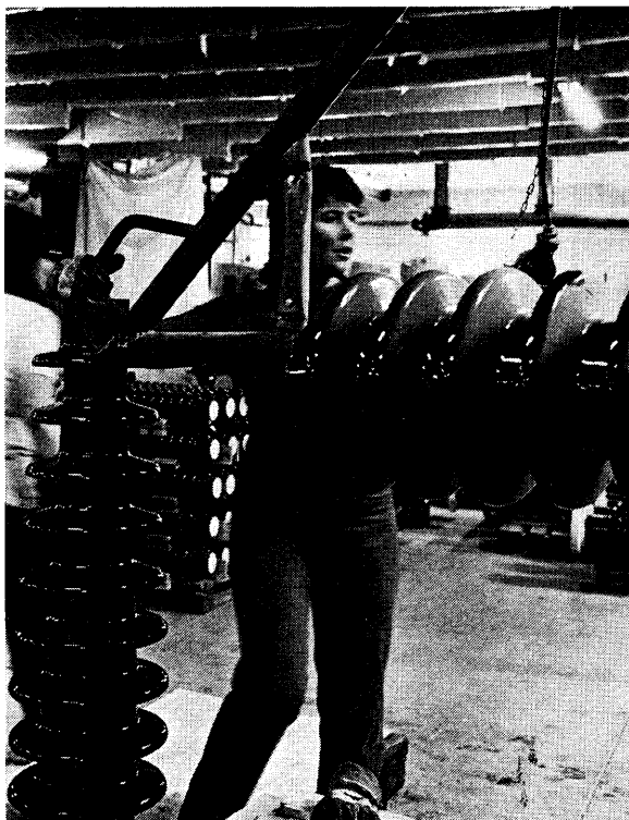
Birgit Julleson sköter maskinen som slipar de här isolatorerna i kortändarna. Den som hon håller i är just färdig-slipad.
